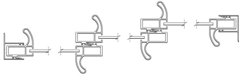
3-løper sett ovenfra STANDARD RETNING
