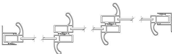
3-løper sett ovenfra STANDARD RETNING
