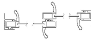
2-løper
