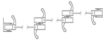
3-løper
