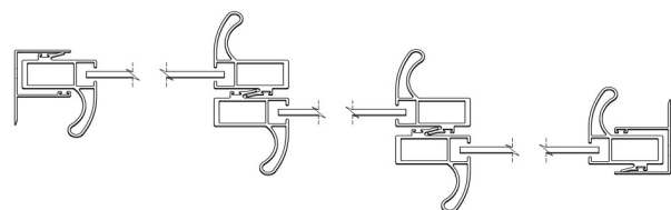
3-løper sett ovenfra SPEILVENDT RETNING
